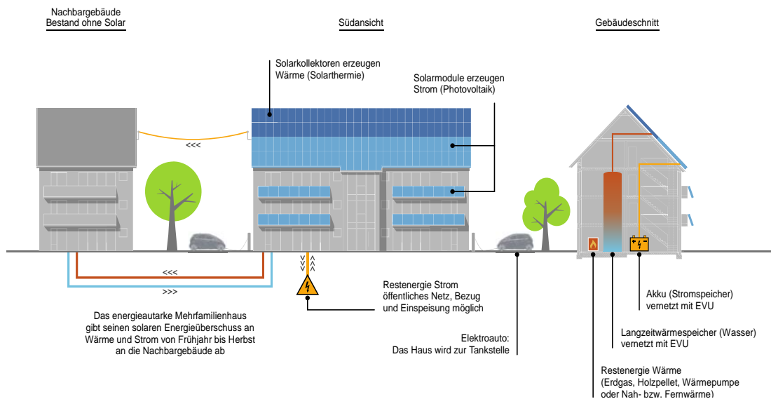
Abb.: Prinzip der vernetzten Energieautarkie, das Solardach bestehend aus Solarthermie- und PV-Modulen sowie schräg montierte PV-Module an der Balkonbrüstung; Positionierung des Langzeitwärmespeichers im Gebäude über mehrere Etagen.
